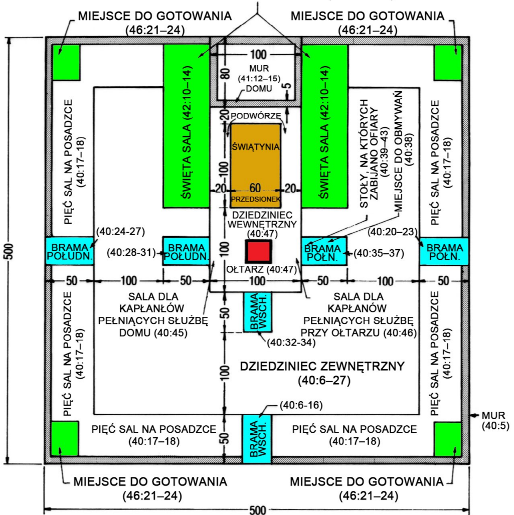
RYSUNEK nr 1: OGÓLNY PLAN ŚWIĄTYNI I DZIEDZIŃCA WEWNĘTRZNEGO ORAZ ZEWNĘTRZNEGO
